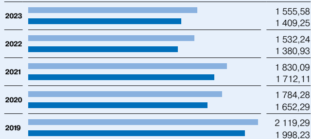
Динамика валовых выбросов в атмосферный воздух в компаниях Группы Газпром, 2019–2023 гг., тыс. т
