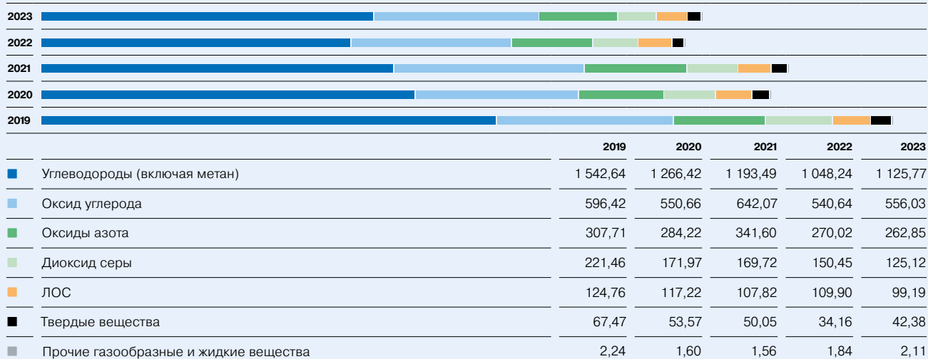
Динамика выбросов основных ЗВ в атмосферный воздух от стационарных источников в Группе Газпром, 2019–2023 гг., тыс. т
