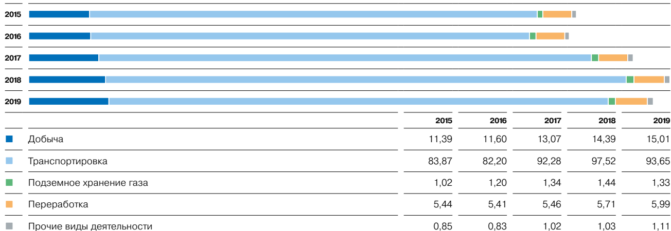
Динамика выбросов ПГ в ПАО «Газпром» по видам деятельности, 2015–2019 гг., млн т CO 2 -экв.
